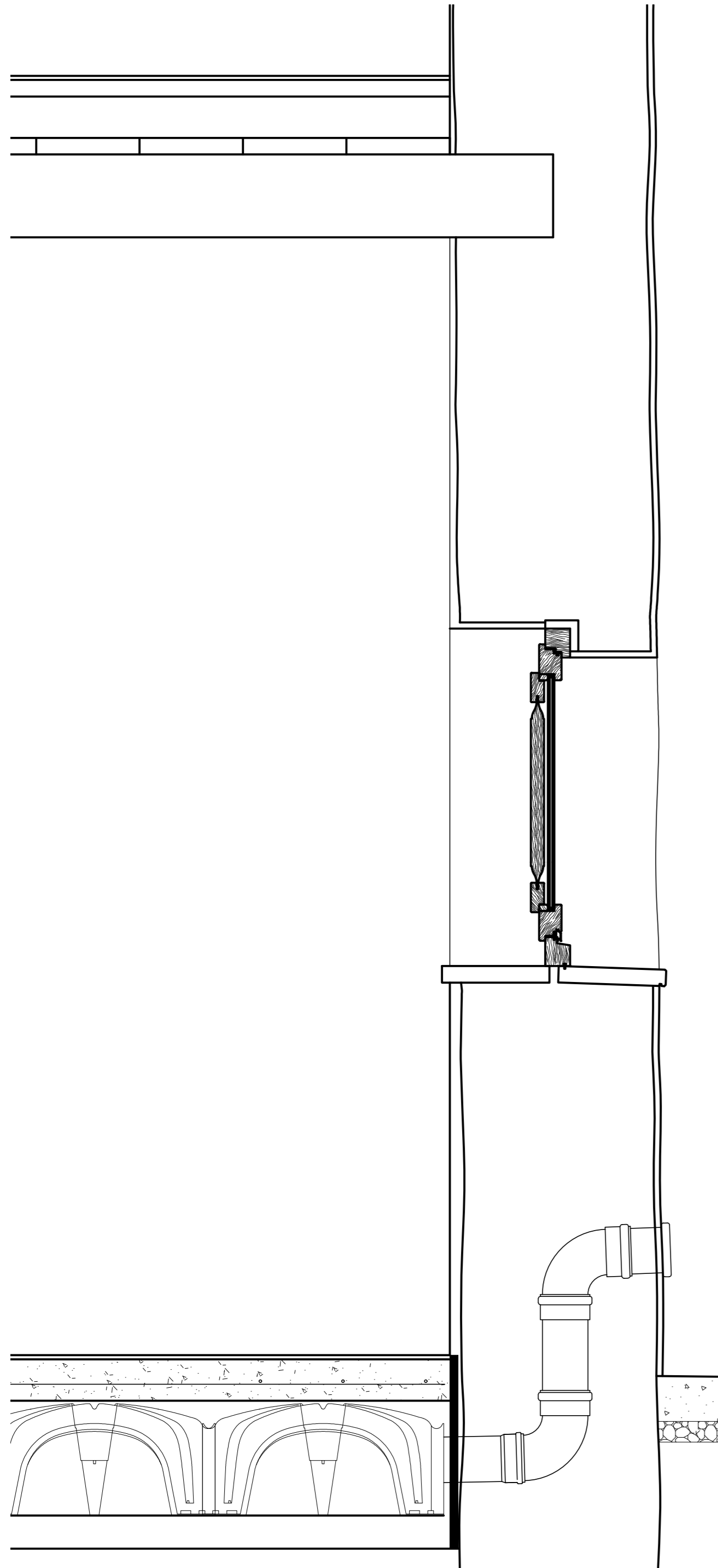
PARTICOLARE COSTRUTTIVO SEZIONE VERTICALE - PROGETTO scala 1:10
